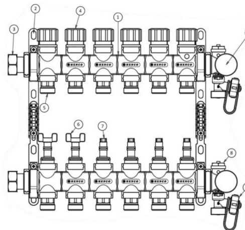
Конструкция коллекторной группы UFH-MDK
